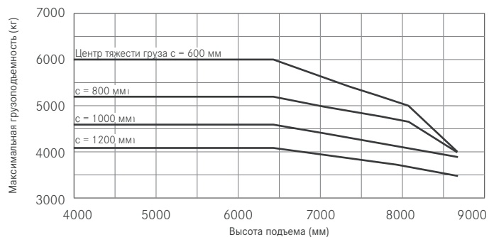
Максимальная грузоподъемность RX 70-60 мачта триплекс – Одинарные шины суперэластик
