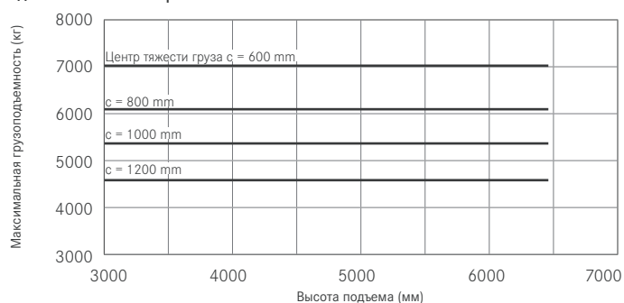
Максимальная грузоподъемность RX 70-70 Телескопическая мачта – сдвоенные шины Superelastic
