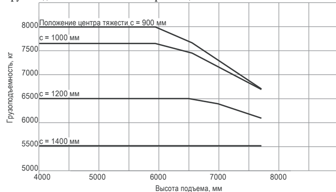
Грузоподъемность RX 60-80/900 с трехсекционной мачтой
