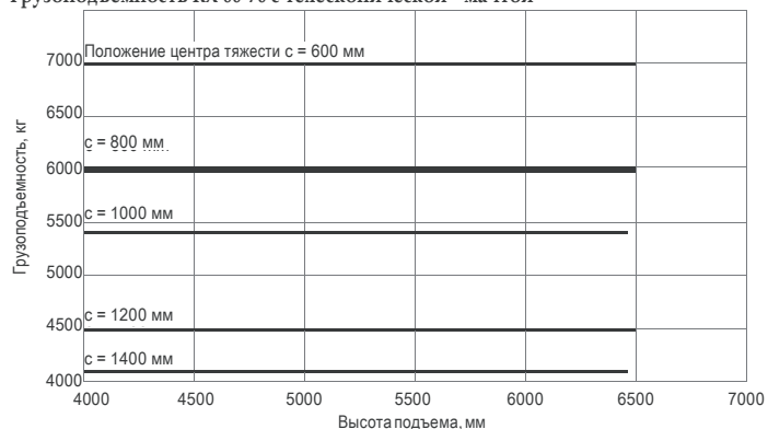
Грузоподъемность RX 60-70 с телескопической мачтой
