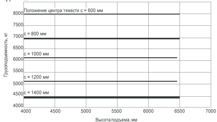
Грузоподъемность RX 60-80 с телескопической мачтой
