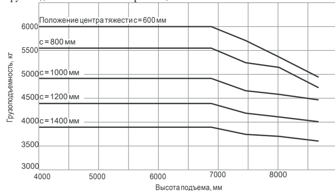
Грузоподъемность RX 60-60 с трехсекционной мачтой
