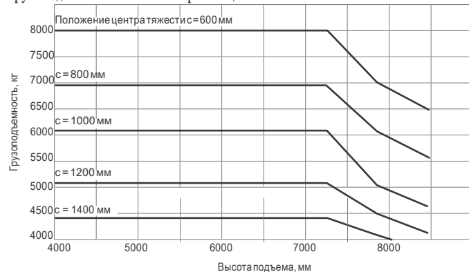
Грузоподъемность RX 60-80 с трехсекционной мачтой
