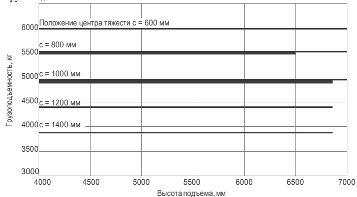
Грузоподъемность RX 60-60 с телескопической мачтой
