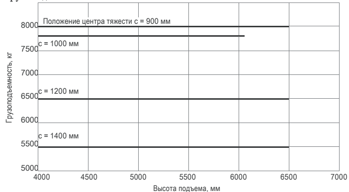
Грузоподъемность RX 60-80/900 с телескопической мачтой
