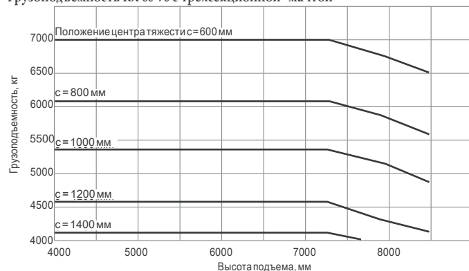
Грузоподъемность RX 60-70 с трехсекционной мачтой
