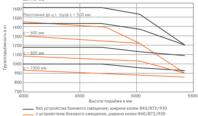
Грузоподъёмности RX 50-16 рама телескоп/NiHo Шины SE
