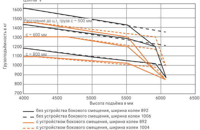
Грузоподъёмности RX 50-16 тройная рама Шины V
