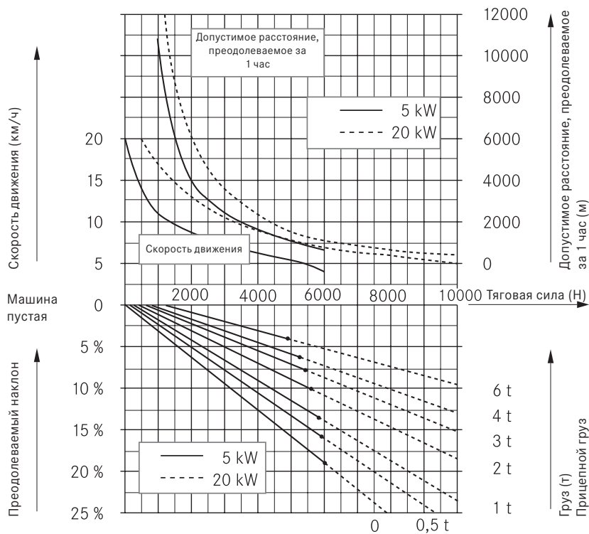
Диаграмма мощности R 08-20
