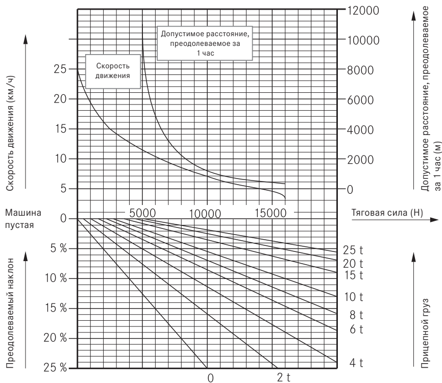
Диаграмма мощности R 07-25
