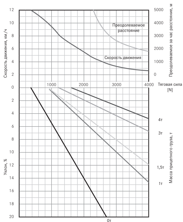
График технических возможностей Kanvan 05.
