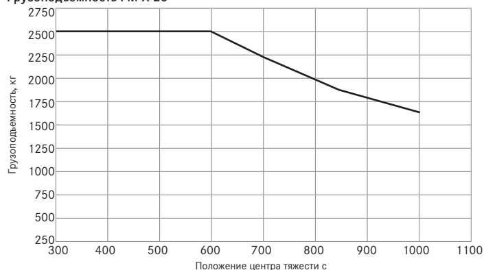
Грузоподъемность FM-X 25
